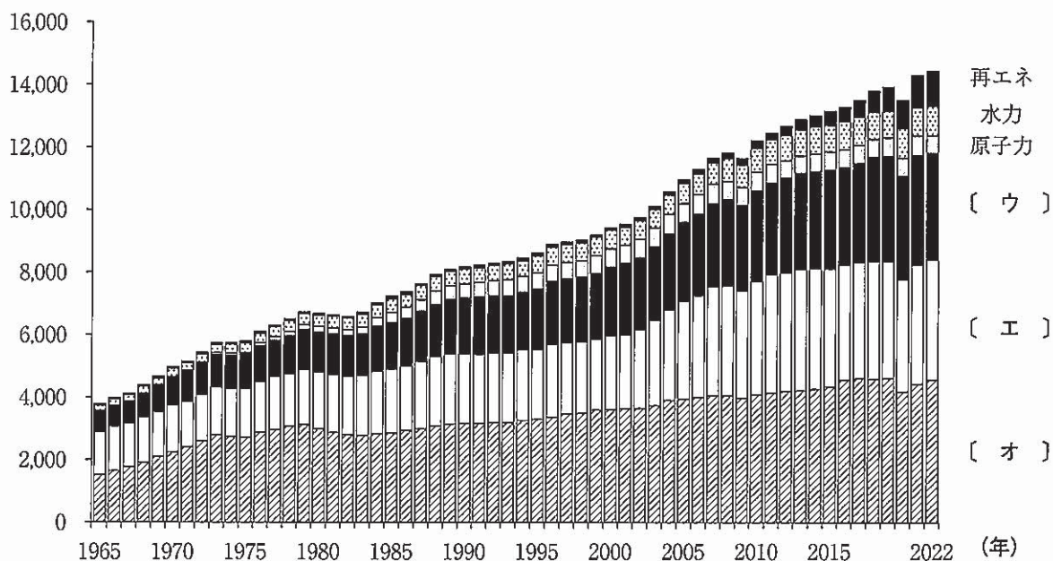
〔図2〕 世界のエネルギー消費の推移（エネルギー源別、一次エネルギー消費）
